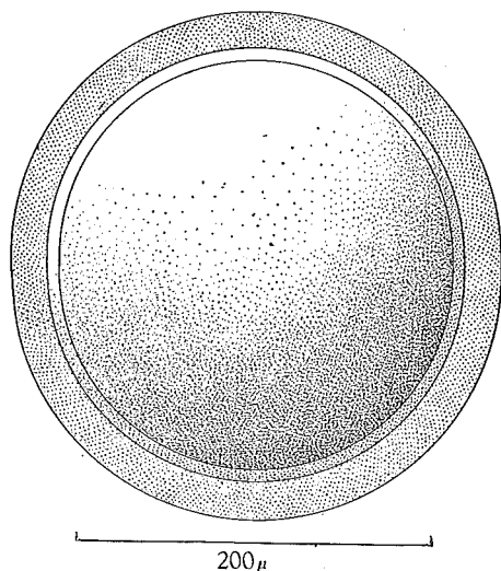
FIG. 25. — Actinocephalus teffli n. sp. Kyste prêt à être expulsé par l'hôte.
