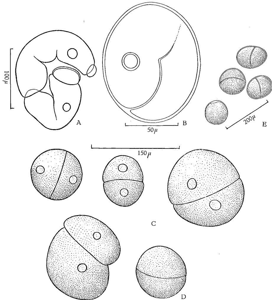
FIG. 20. — Gregarina crenata (BHATIA et SETNA.)
