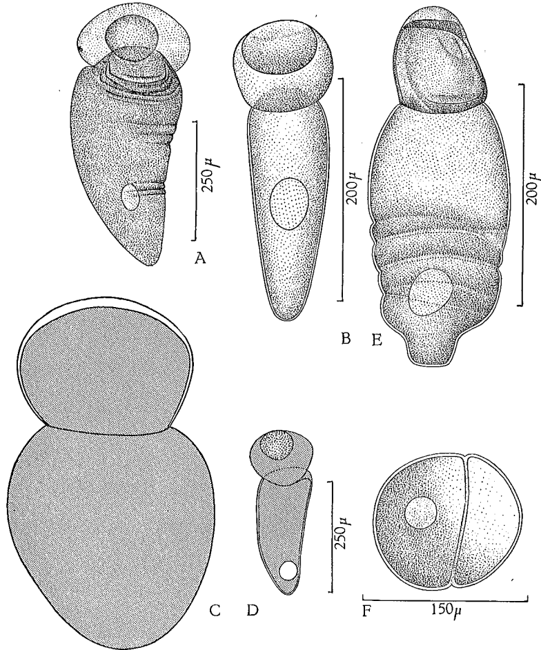
FIG. 24. — Actinocephalus tefli n. sp.
