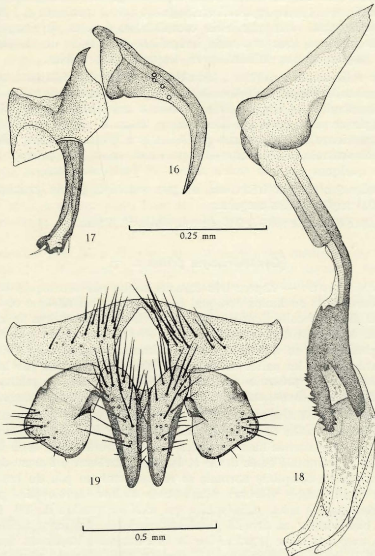
FIG. 16-19. — Gynandromyia saegeri n. sp., type (Gy 9).
