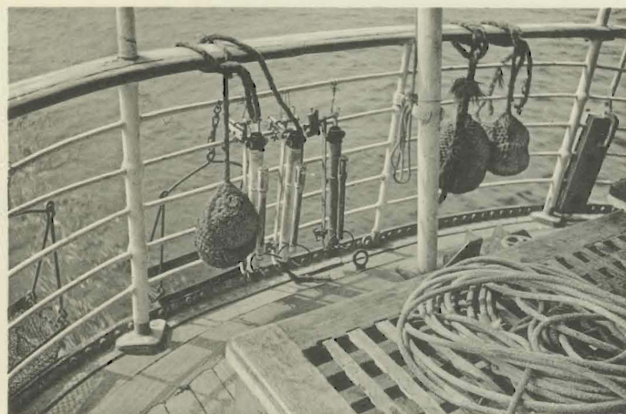
Fig. 3. — Bouteilles de NANSEN utilisées pour la mesure de la température et la prise d'échantillons d'eau en profondeur. C.
