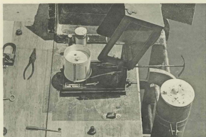
Fig. 5. — Limnigraphe enregistreur du port d'Albertville. C.
