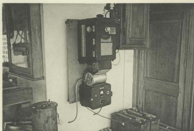
Fig. 6. — L'échosondeur enregistreur HUGHES M. S. 19 , utilisé pour l'étude du relief du fond du lac. C.
